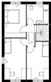
Obergeschoss TOP 2.1
